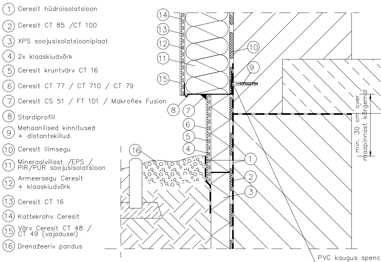
Joonis 3. Ceresit Ceretherm SILS süsteemi sokli ja panduse lõige.
