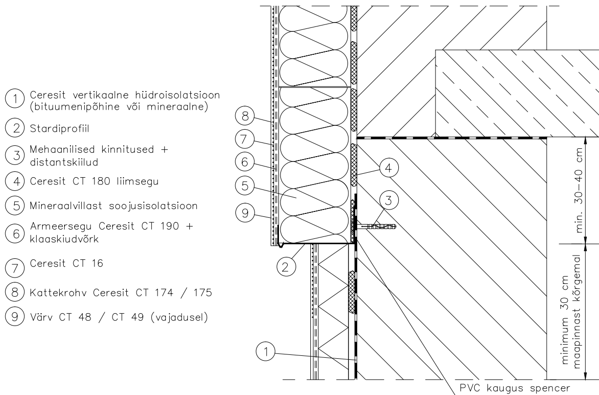
Joonis 2. Ceresit Ceretherm SILS mineraalvilla ühendus sokliga.
